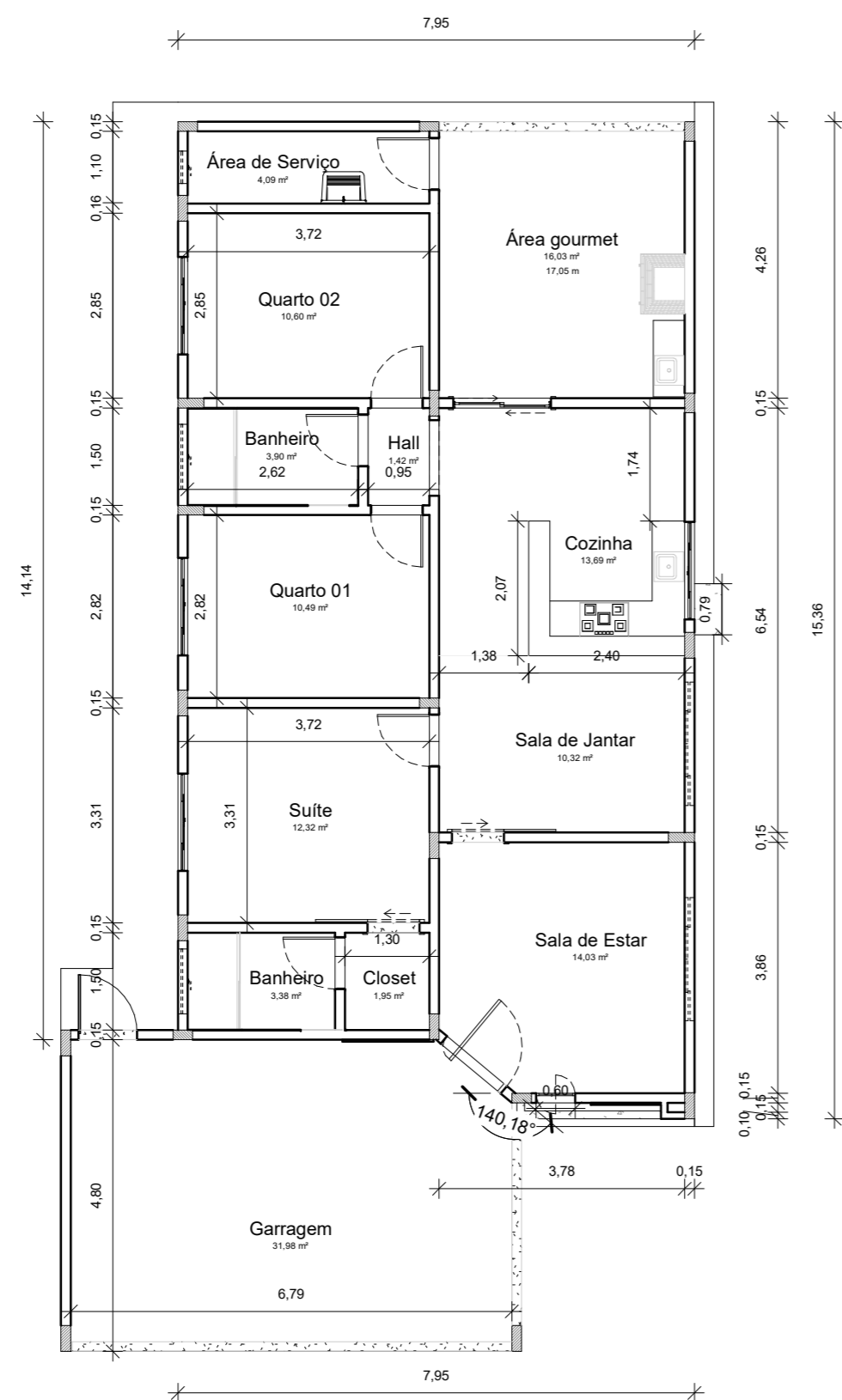
3 PLANTA BAIXA - TÉRREO Escala: 1 : 100
