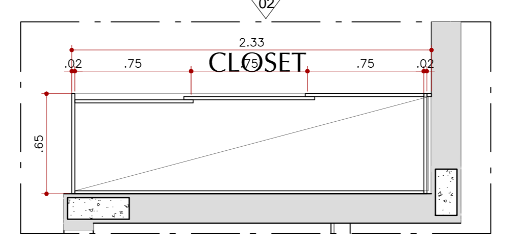
PLANTA CLOSET ESC. 1:25
