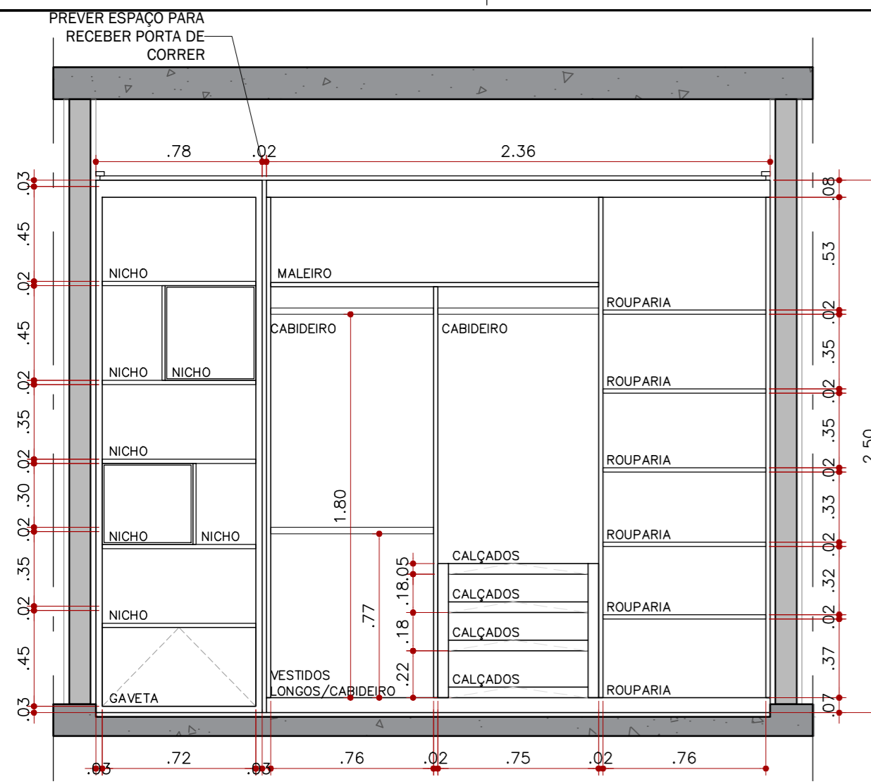
ELEVÇÃO 01 CLOSET ESC. 1:25
