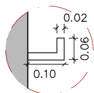
DET.01 1:10
