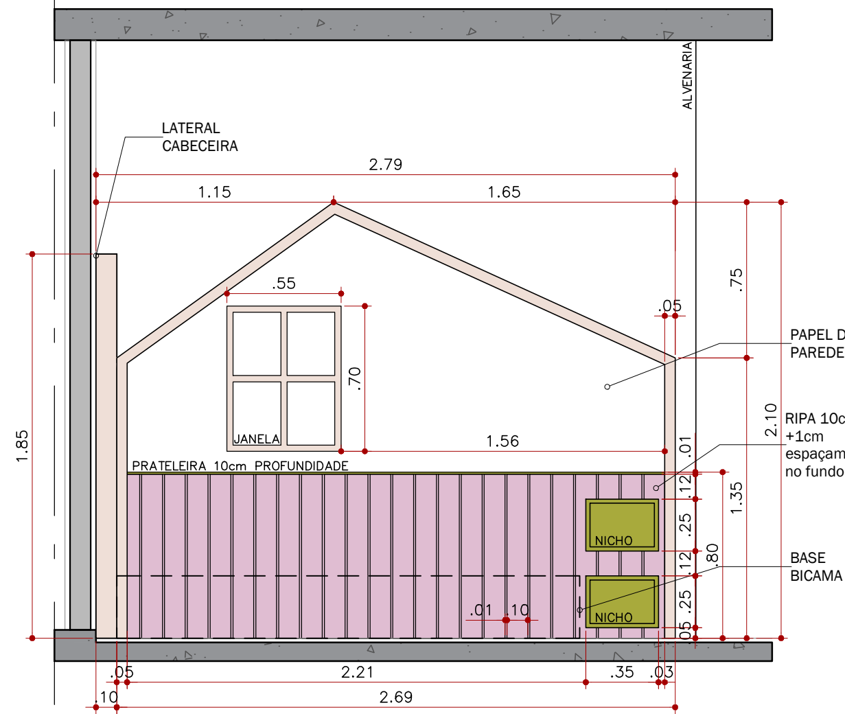
ELEVAÇÃO 05 CASINHA ISIS ESC. 1:25
