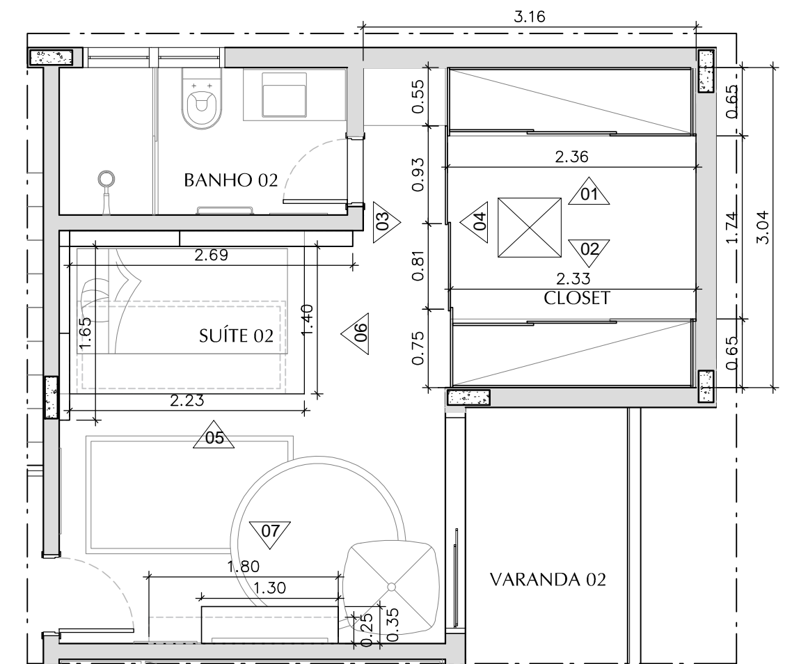
PLANTA LOCAÇÃO SUÍTE ISIS ESC. 1:50
