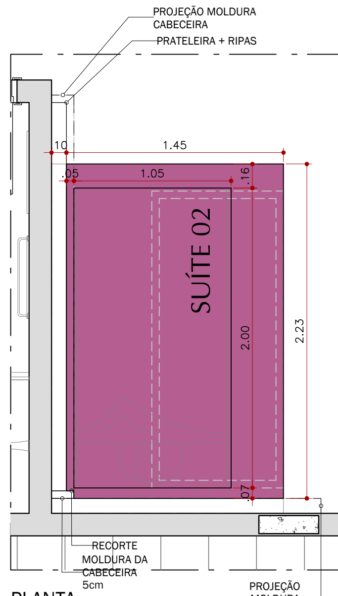
PLANTA BASE BICAMA ESC. 1:25
