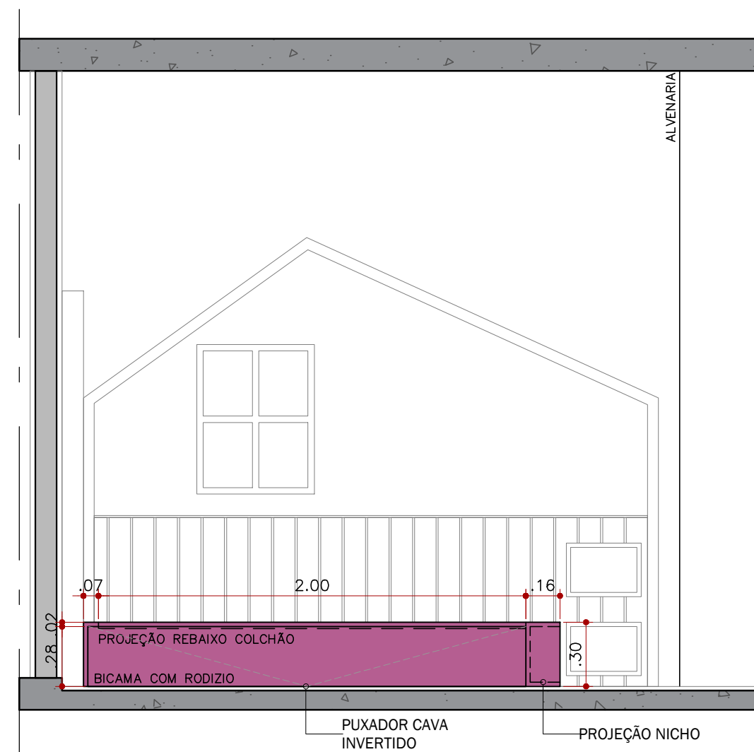
ELEVAÇÃO 05 BASE BICAMA ESC. 1:25
