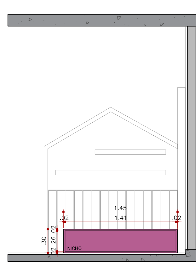
ELEVAÇÃO 06 BASE BICAMA ESC. 1:25
