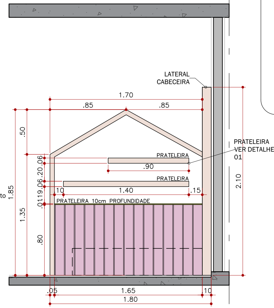
ELEVAÇÃO 06 CASINHA ISIS ESC. 1:25
