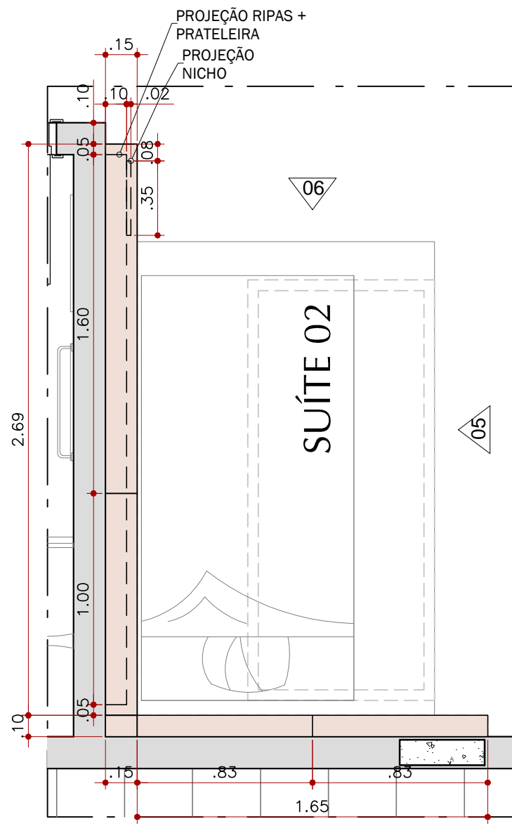
PLANTA CASINHA ISIS ESC. 1:25
