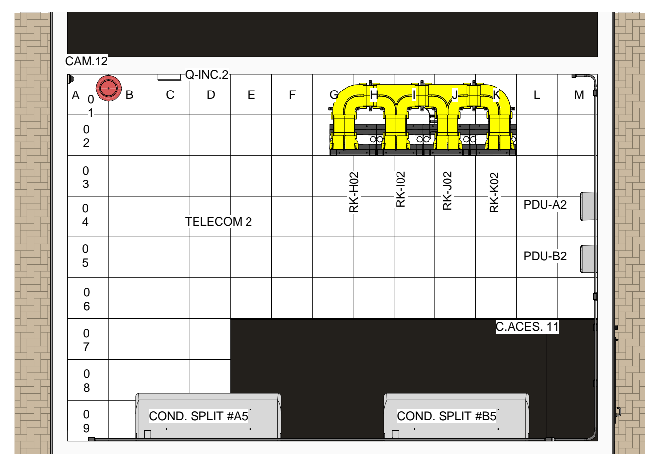
4 TELECOM 2 1 : 50
