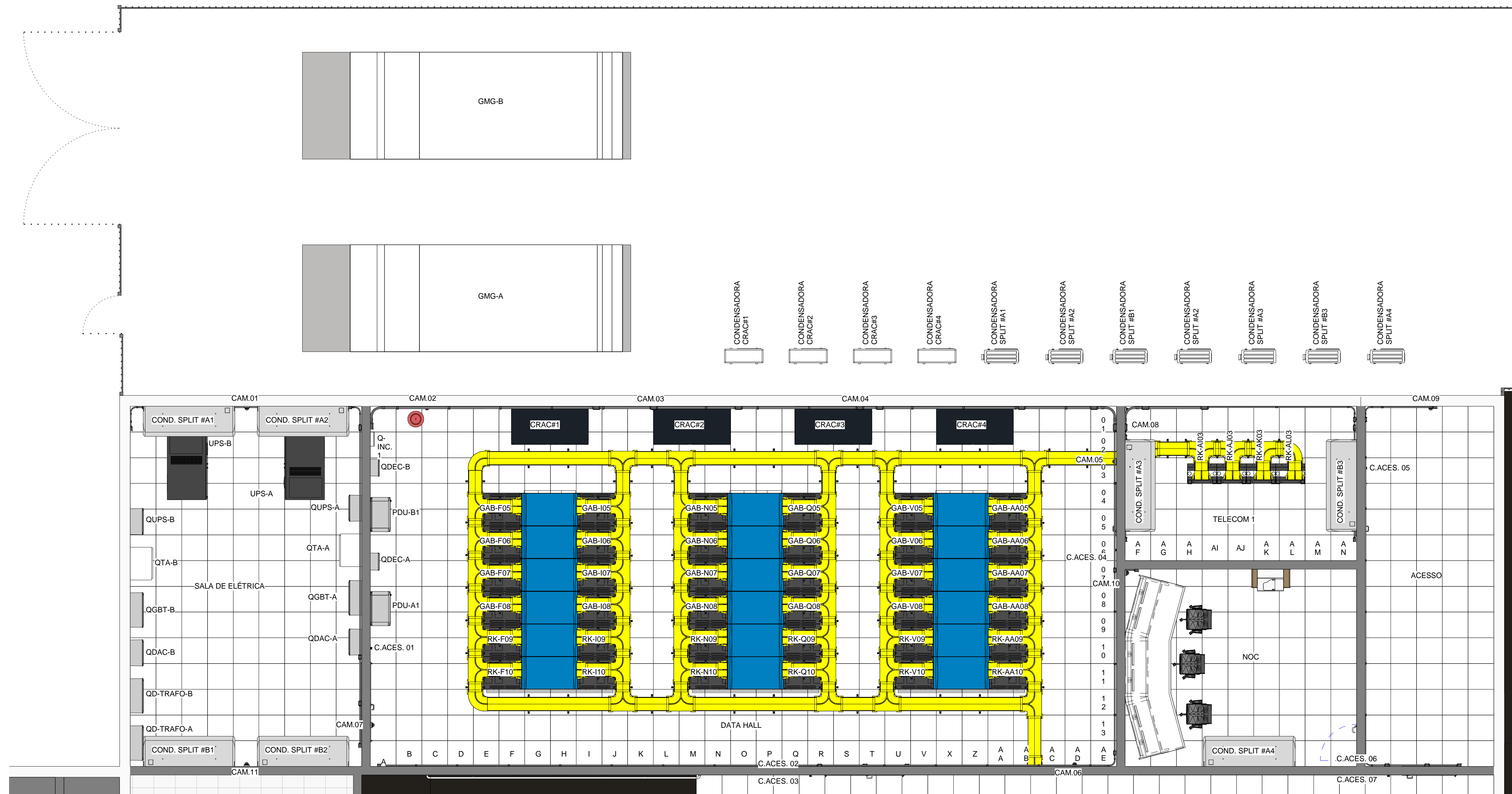
1 DATA CENTER 1 : 50
