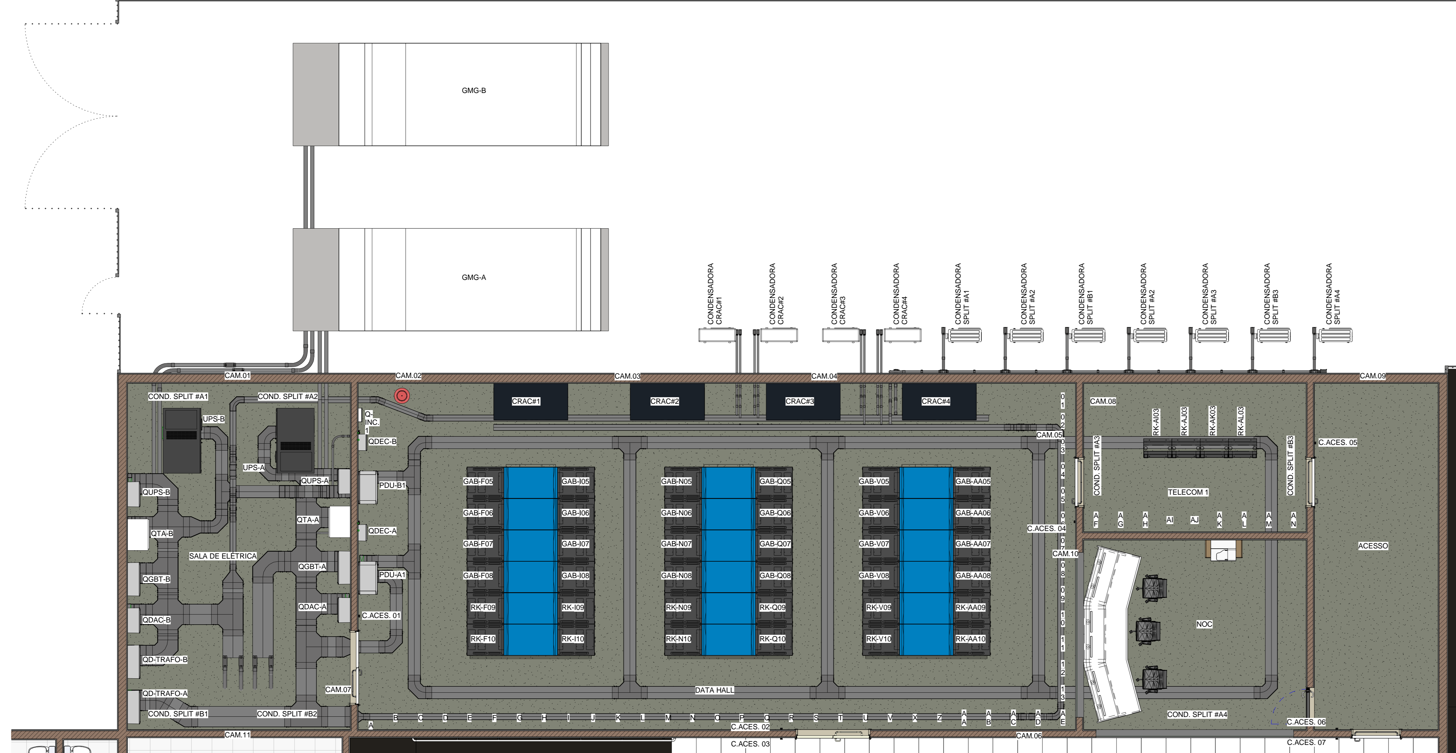
1 DATA CENTER 1 : 50
