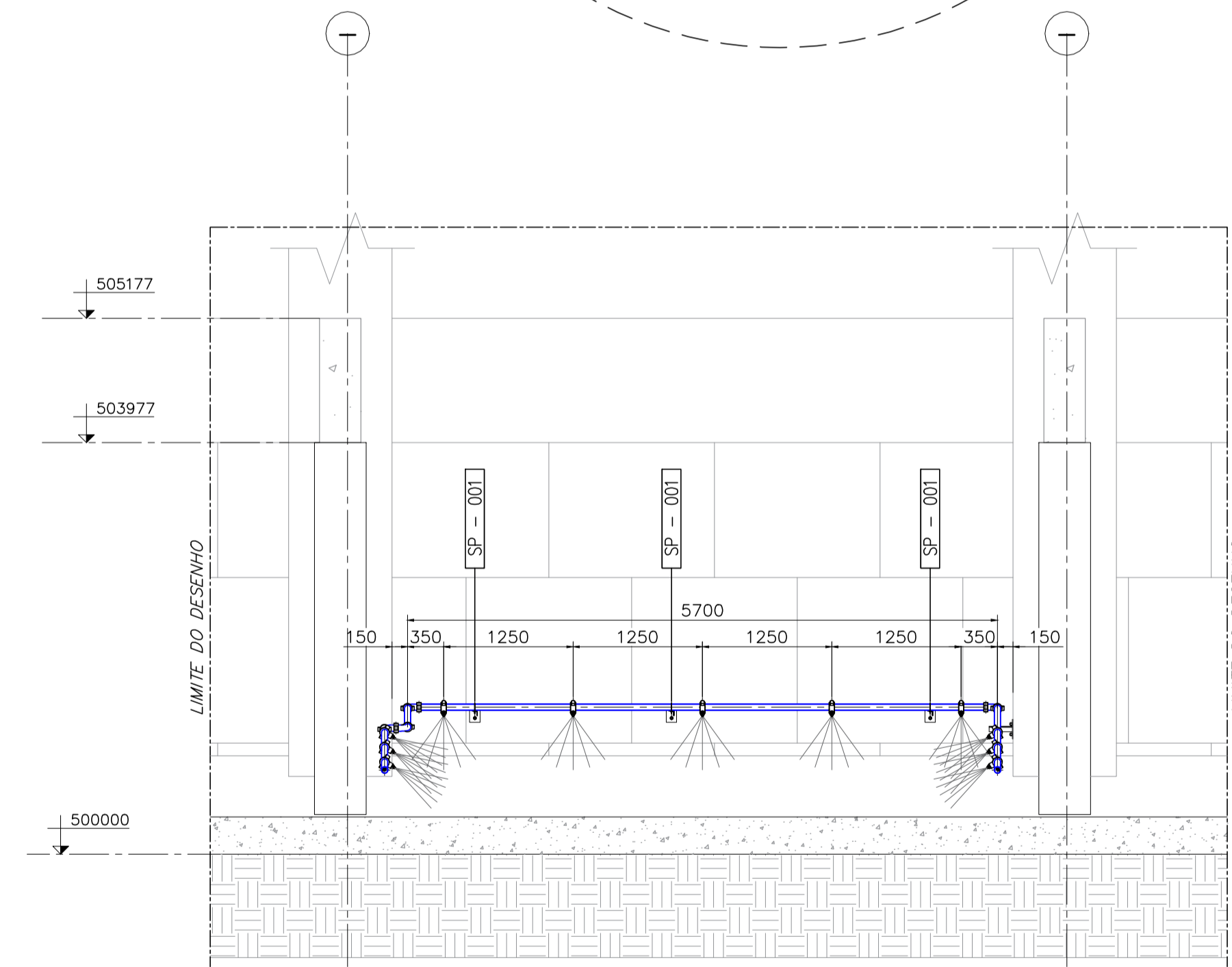
CORTE C-C ESCALA: 1:50
