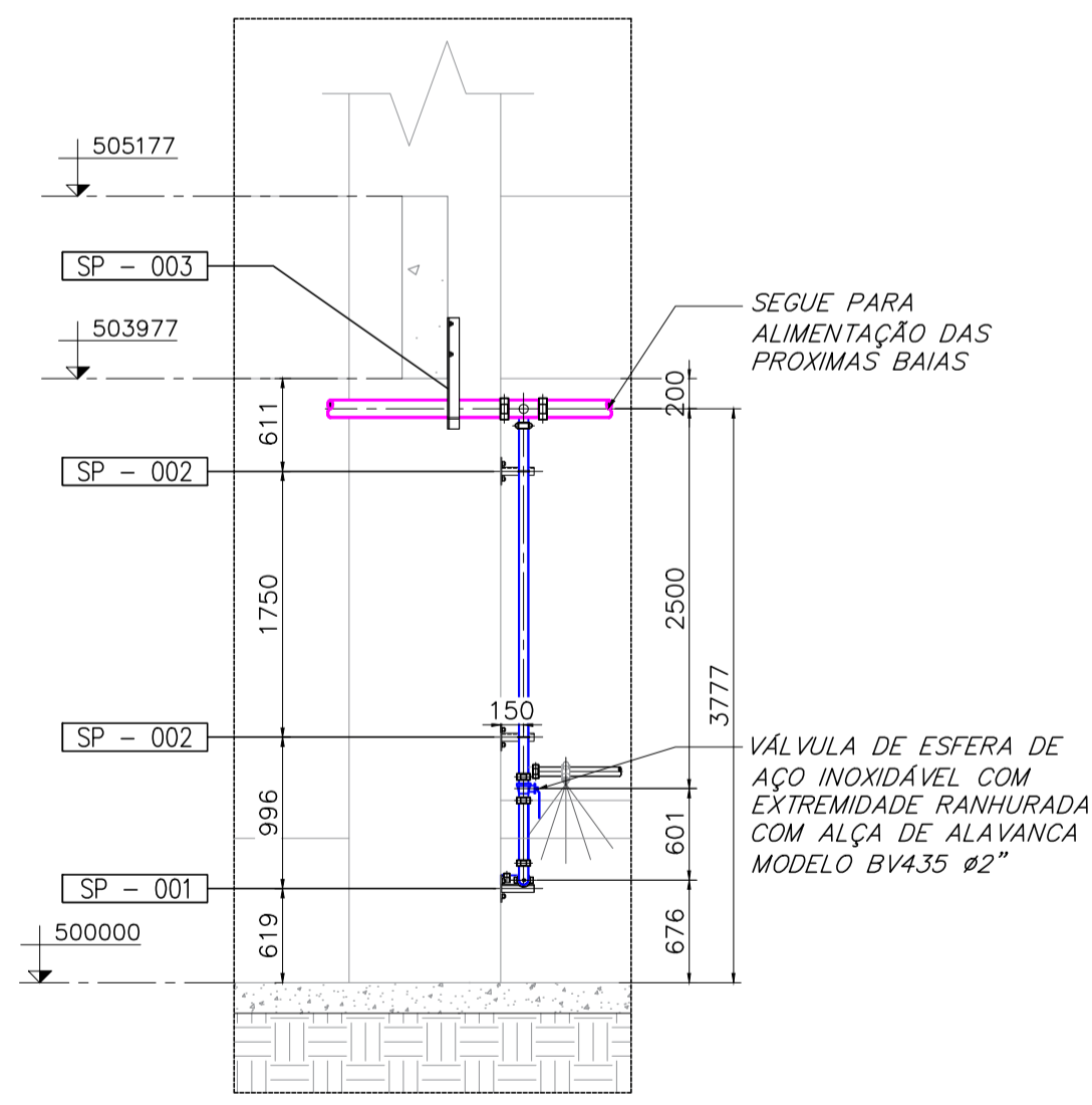
DET. 01 ESCALA: 1:50
